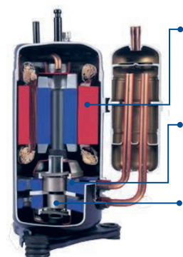
Двухроторный инверторный компрессор
